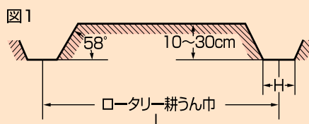
図1は1畦1耕程 図2は片側セット にて連接広巾畦が できます。
